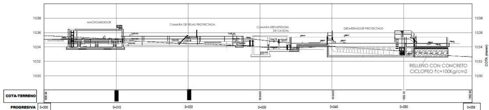
PERFIL LONGITUDINAL PROG: 0+000 A 0+059 Esc.: 1/100
